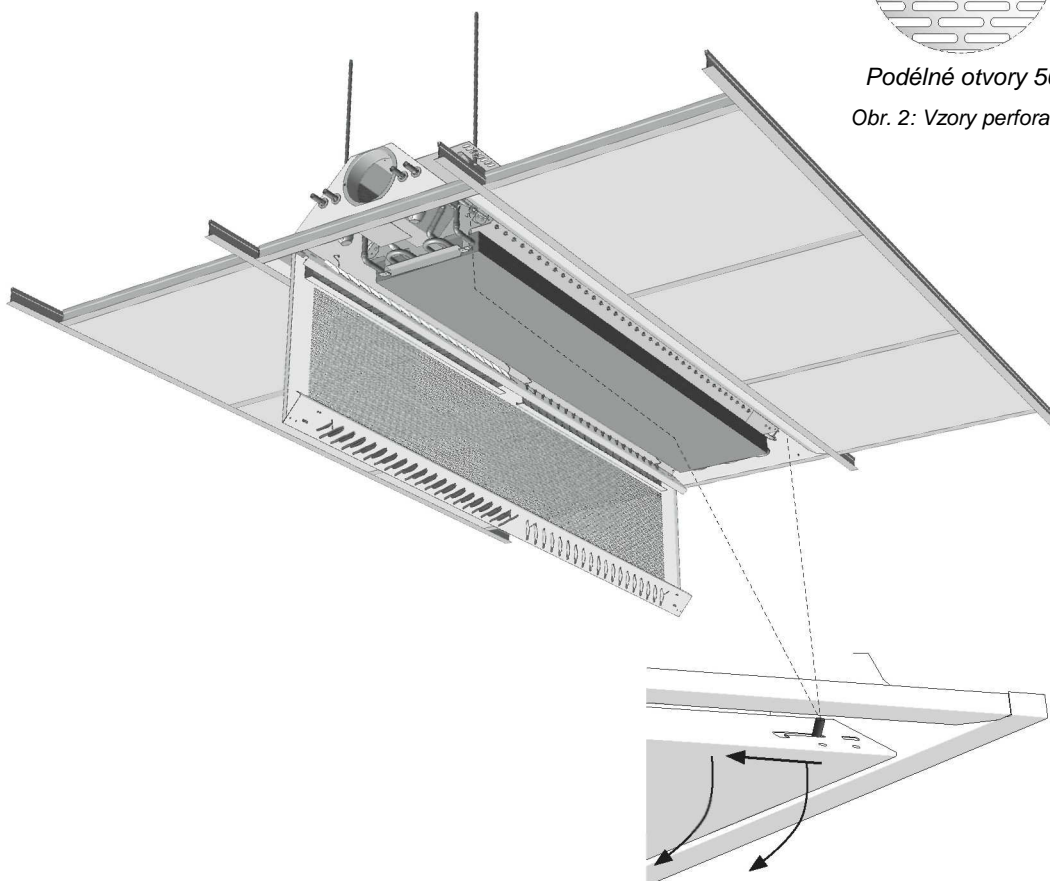
Obr. 3: Po sklopení nebo odmontování čelního panelu je zespona výměník přístupný pro čištění. Na obrázku je také vidět systém AirGuide, který se dodává jako volitelná výbava trámu jako alternativa systému směrových trysek.
