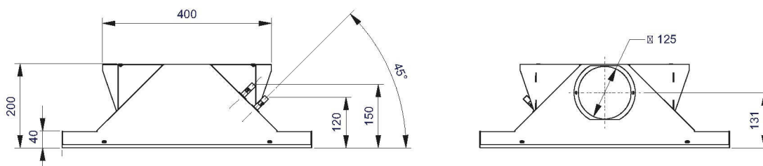
Obr. 7: Možné varianty připojení chladicí a topné vody k trámu Premax I-60-A
