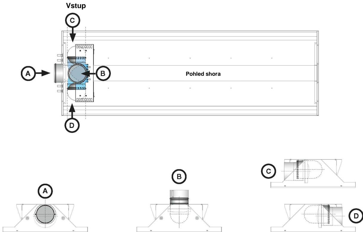
Obr 1: Pro připojení typu A je trám Premax dodán se standardním připojovacím hrdlem Lindab (NPU-125). Pro připojení typu B, C a D je součástí dodávky trámu koleno Lindab (BU 90°).
