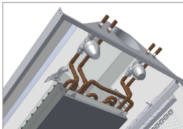
Figúre 6. Ilustrační obrázek umístění regulačního ventilu a servopohonu uvnitř chladicího trámu , A1 příklad, Premax (volitelné příslušenství).
