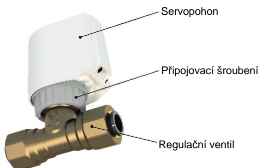
Obr. 5: Regulační ventil LinFlow-S s namontovaným servopohonem.
