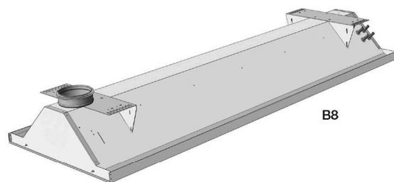
Obr. 4: Příklad nejčastějších variant A a B připojení přívodu vzduchu k chladícím trámům Premax.
