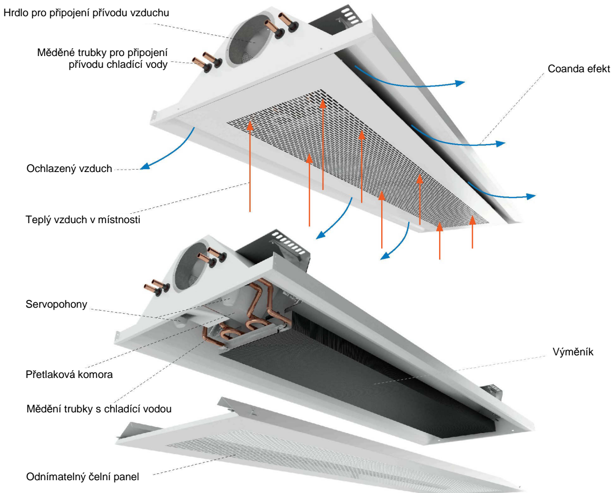
Obr. 1: Chladicí trám Premax - využití principu indukce
